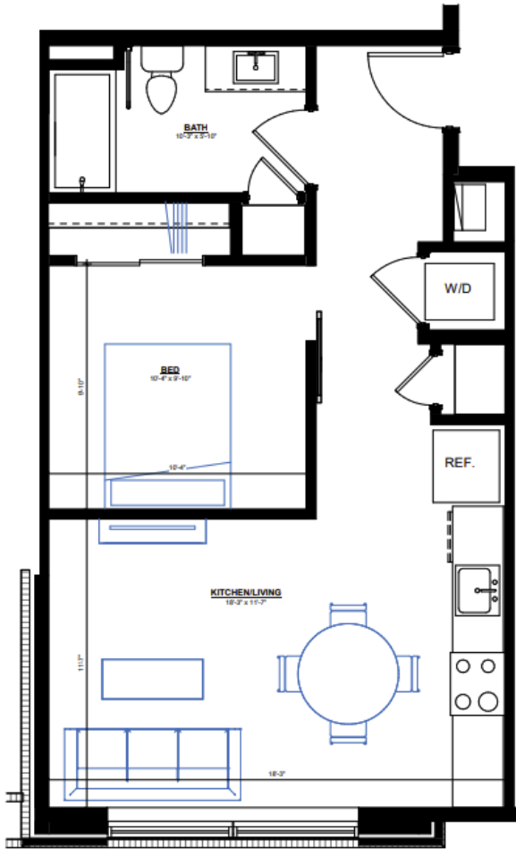
1 SUITE x04, x10 SCALE: 1/2" = 1'-0"
