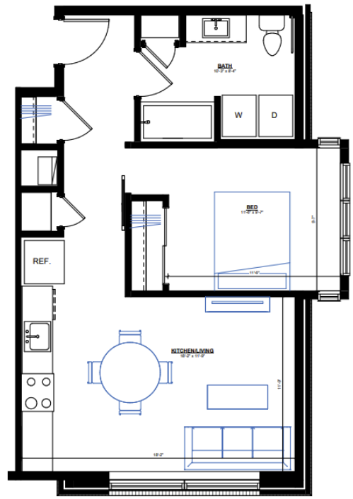
1 SUITE x02 SCALE: 1/2" = 1'-0"
