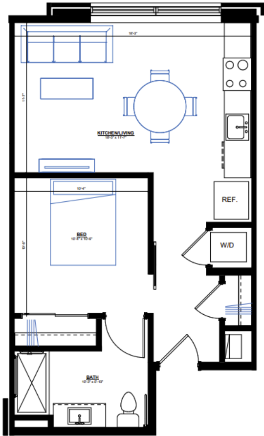
1 SUITE x03 SCALE: 1/2" = 1'-0"
