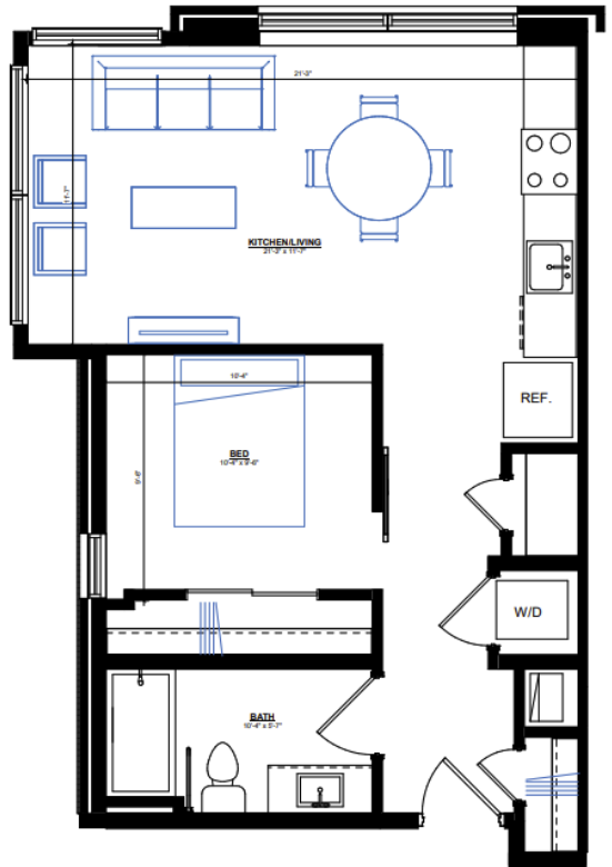
1 SUITE 111 SCALE: 1/2" = 1'-0"
