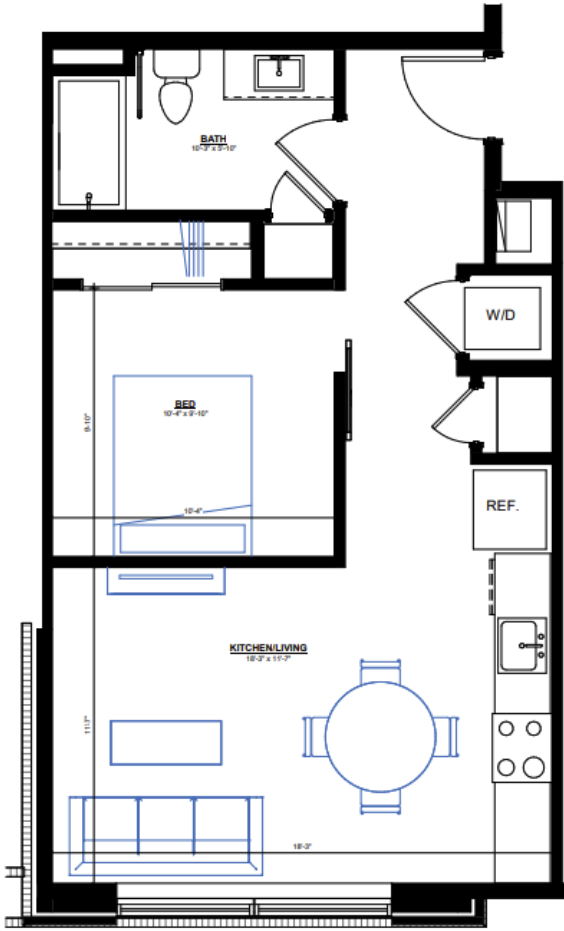
1 SUITE x04, x10 SCALE: 1/2" = 1'-0"
